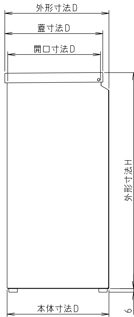
側面図
