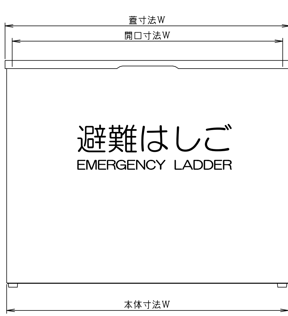
正面図
