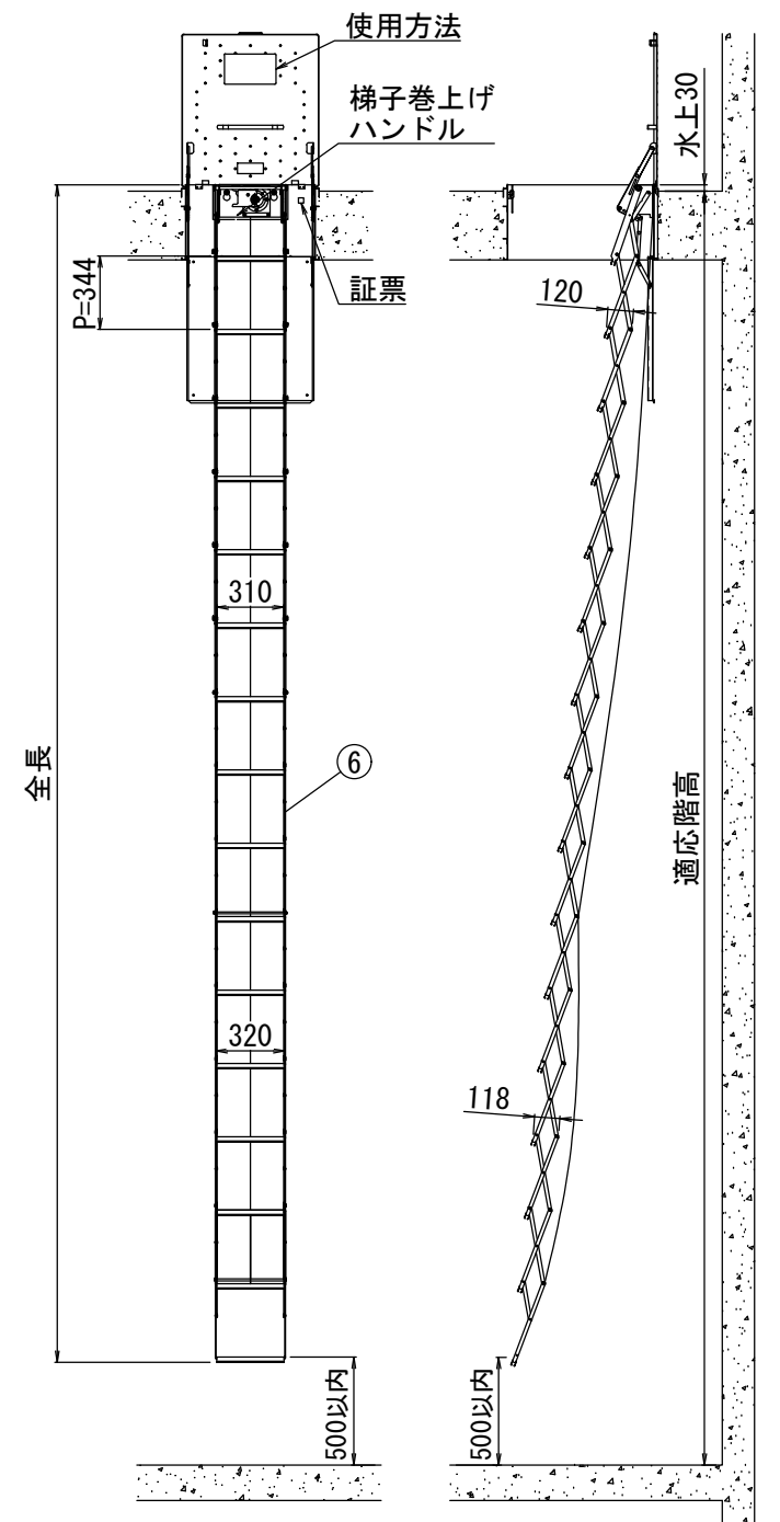
縮尺(1:40)
