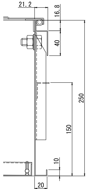
吊元詳細(1:3)
