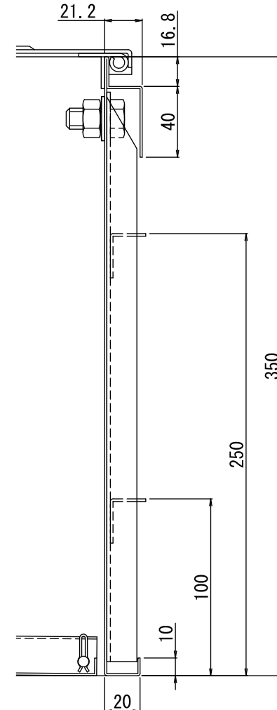
吊元詳細 (1:3)
